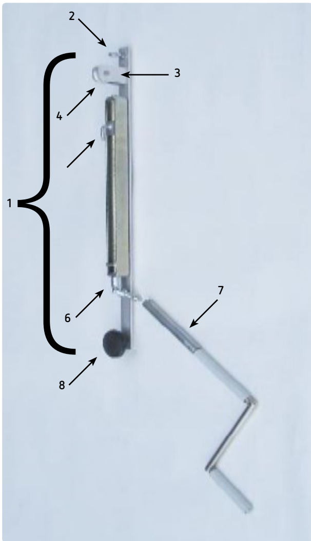
Mechanikschieber
