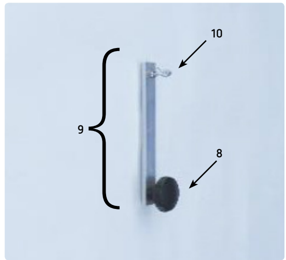
Gegenschieber (Haken-Schiebe-Element)
