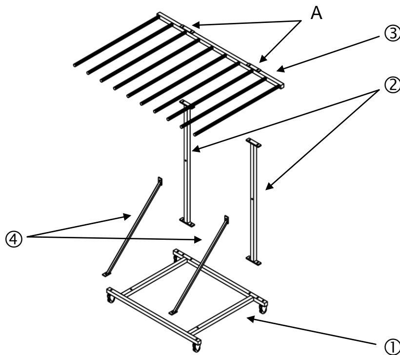
Abb. 2: Explosionszeichnung
