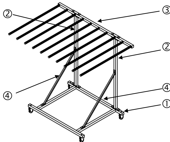
Abb. 1: Mattentransportwagen
